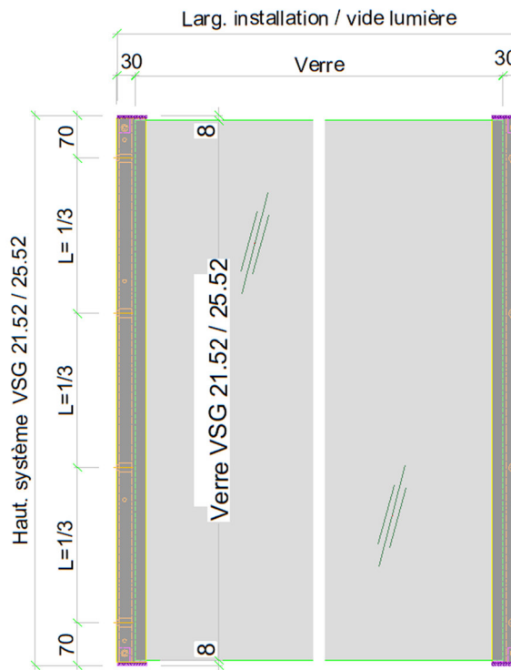
Montage en applique "V" VSG type 21-4 / 25-4
