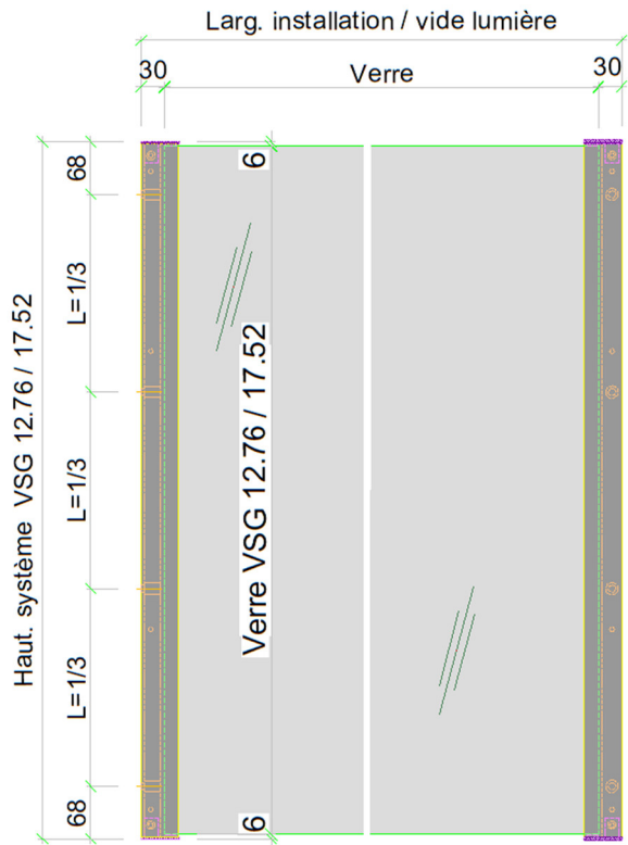
Montage en embrasure "H" VSG type 12-2 / 17-4
