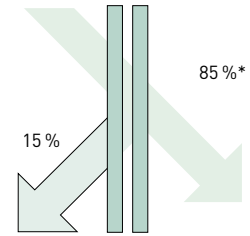
Wärmeschutzisolierglas mit Low-E, ohne Luxar U_v = 1.1 \text{ W/m}^2\text{K}
